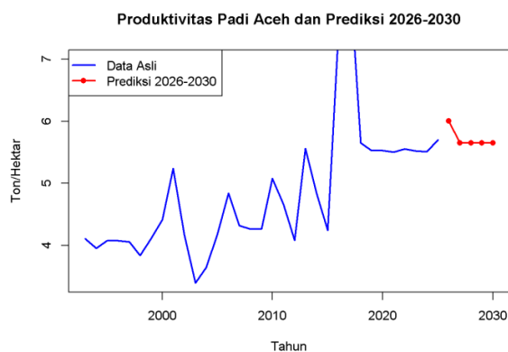
Gambar 4.7 Forecast Produktivitas Padi di Provinsi Aceh Tahun 2026-2030
