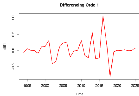
Gambar 4.2 Plot data Produktivitas Padi Provinsi Aceh tahun 1992-2025 Setelah Transformasi dan Differencing
