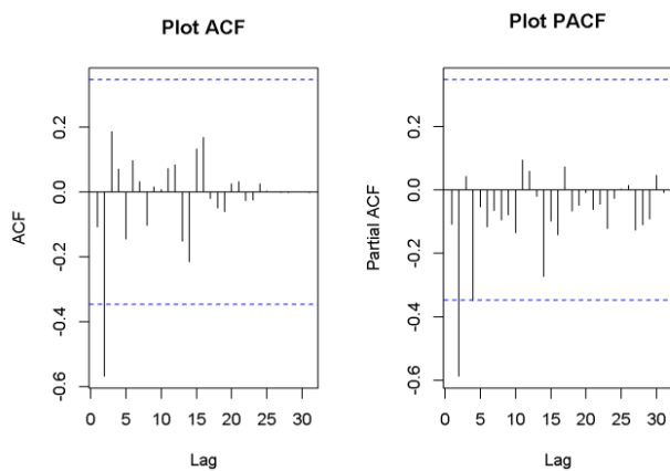
Gambar 4.3 Plot ACF dan PACF Setelah Dilakukan Differencing
