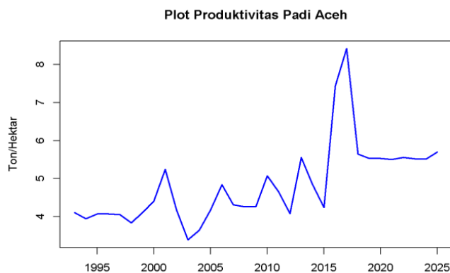
Gambar 4.1 Plot data Produktivitas Padi Provinsi Aceh tahun 1992-2025
